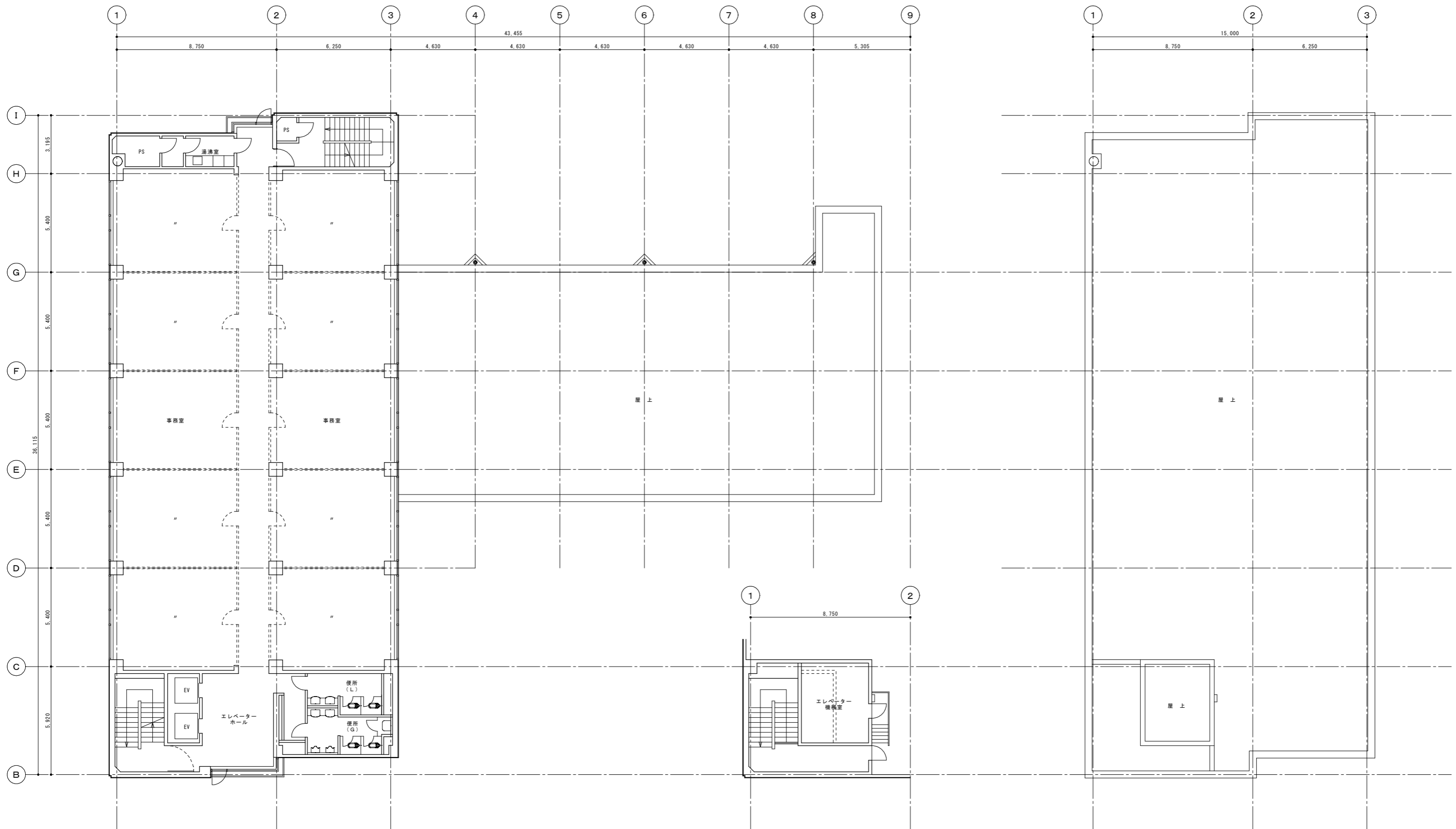
3～7階平面図
